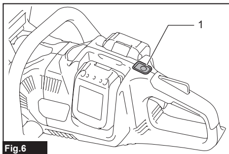
Fig.6 ► 1. Interrupteur d'alimentation secteur
